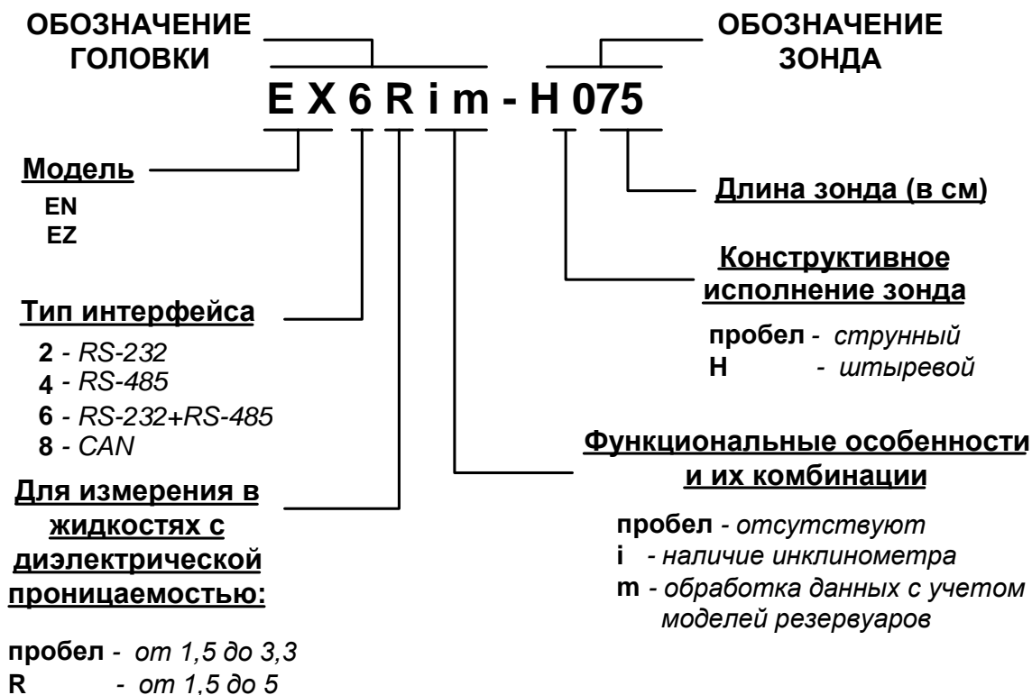
Рис. 1.3 – Обозначение датчиков
