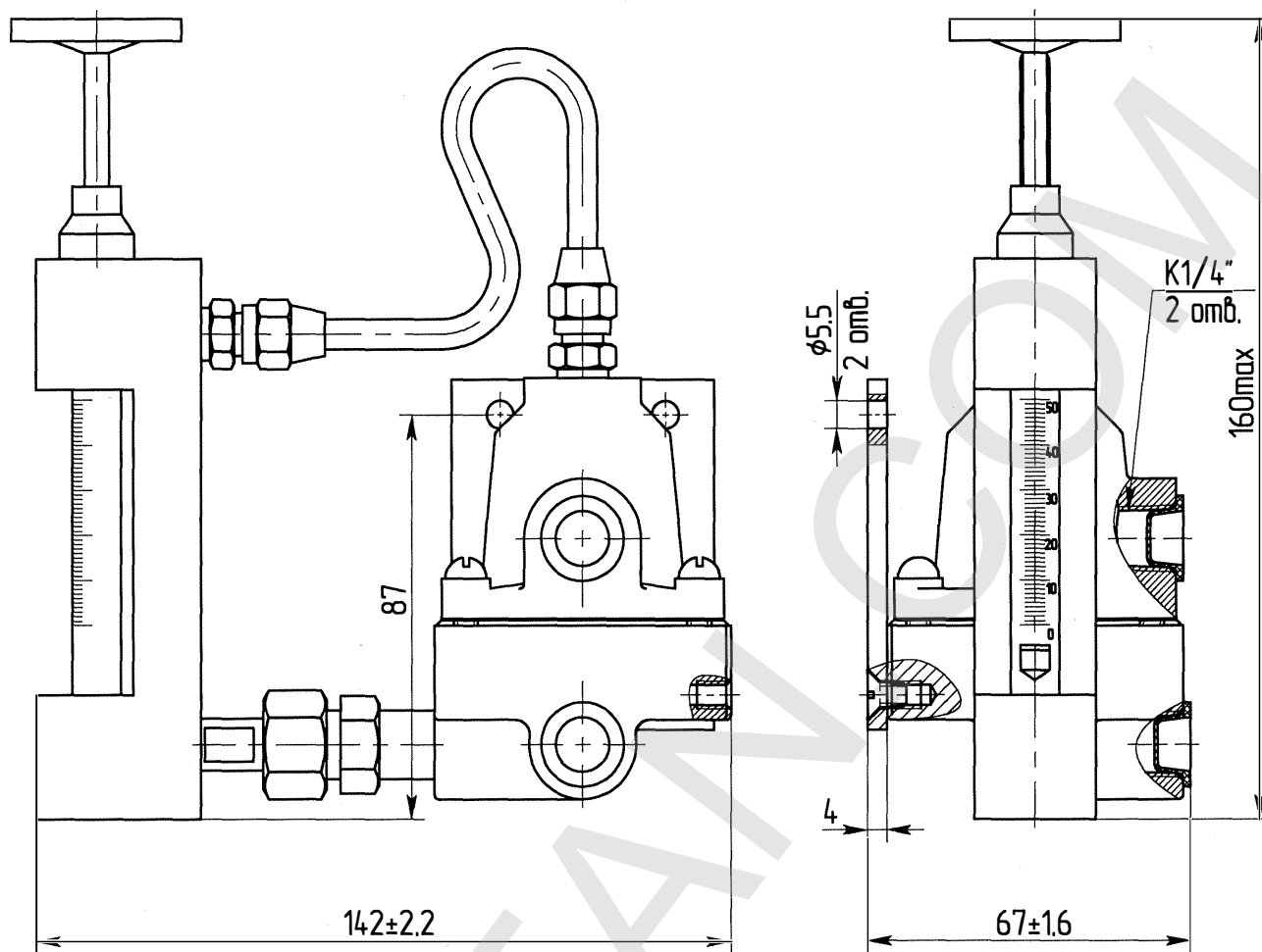
Рисунок А2: Габаритные и присоединительные размеры регулятора PPB-1.
