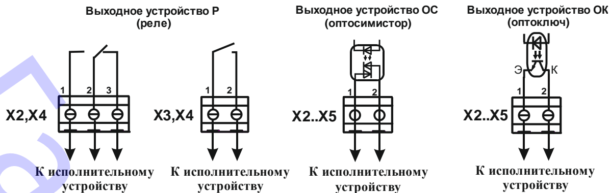
Рисунок 2 – Схемы подключения различных выходных устройств
